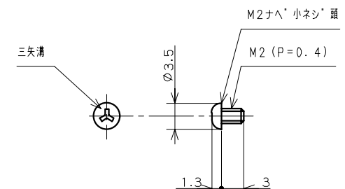
特殊ネジ: ミツ矢詳細
