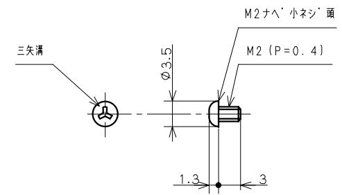
特殊ネジ: ミツ矢詳細
